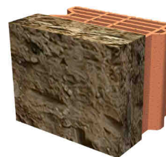
Blocco denominato "EUROBRICK® BIO COMPLETAMENTO", dimensioni nominali 235 x 200 x 190 mm
